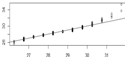
Fig. 4. The q-q plot of A-SD data.
